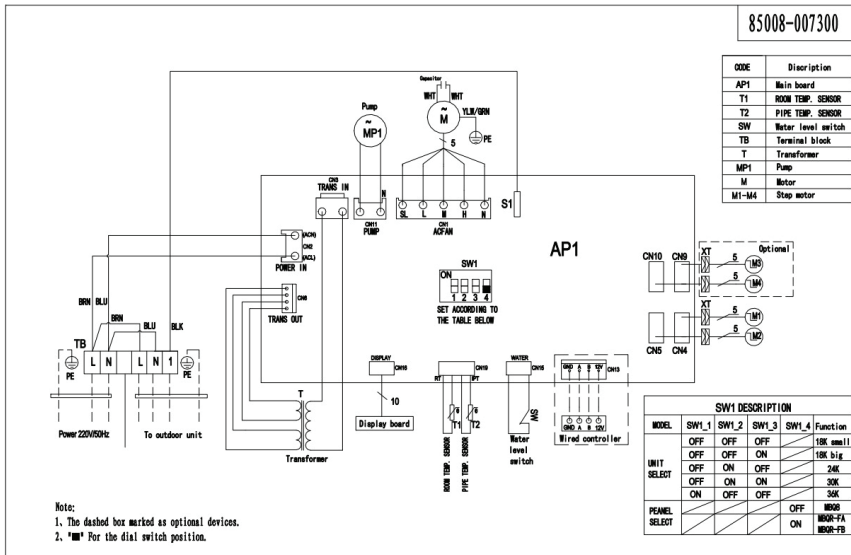
Схема для для внутренних блоков (модель LCAC-24TCI/LCAC-36TCI)
