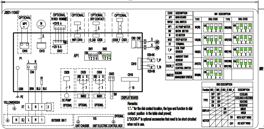
Схема для для внутренних блоков (модель LCAC-18TCI)
